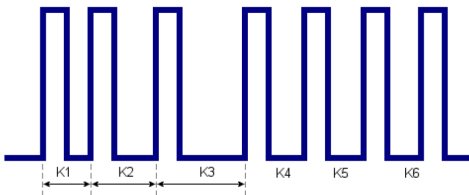
Wykres modułacji PPM w czasie
