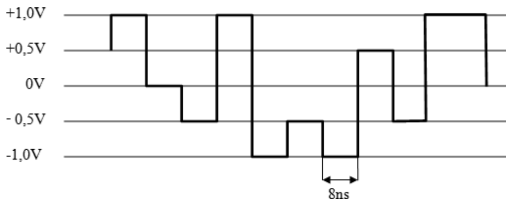
Wykres modułacji PAM w czasie
