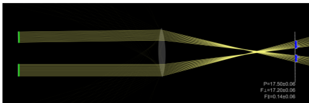
Sytuacja kiedy obraz jest wyostrowiony przed matrycą
