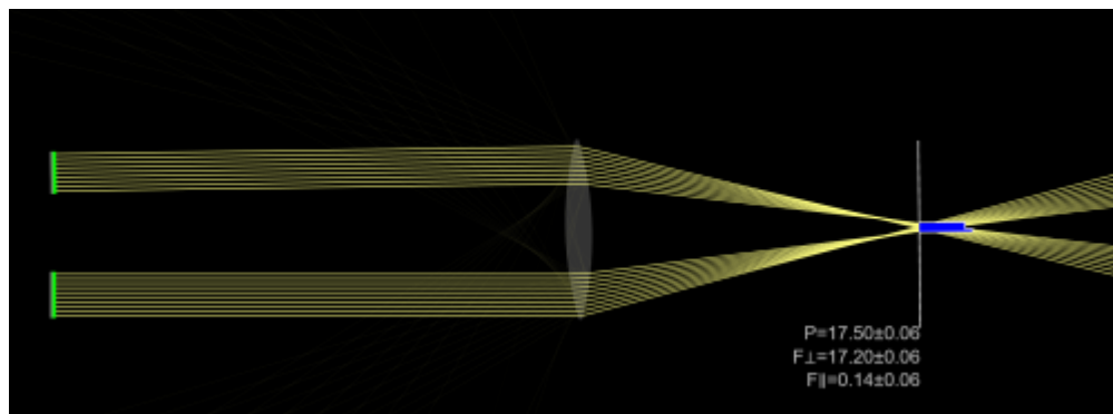
Sytuacja w której obraz jest wyostrowiony na matrycy
