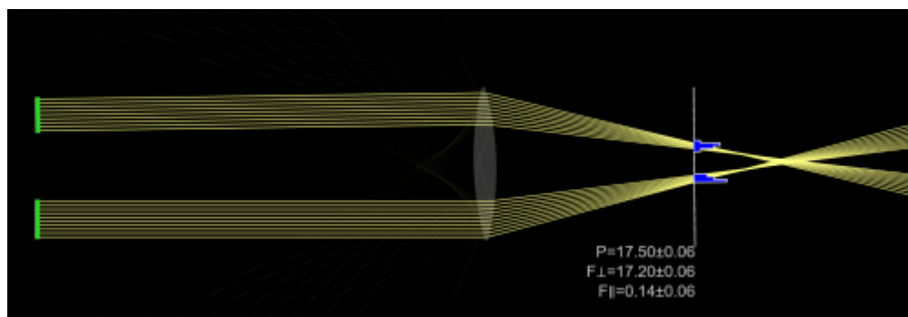
Sytuacja w której obraz jest wyostrowiony za matrycą
